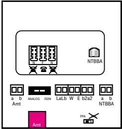
Abb. 1: T-DSL Splitter bis Baureihe 12/2001
