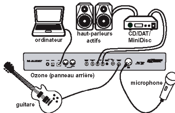
Configuration typique 2
