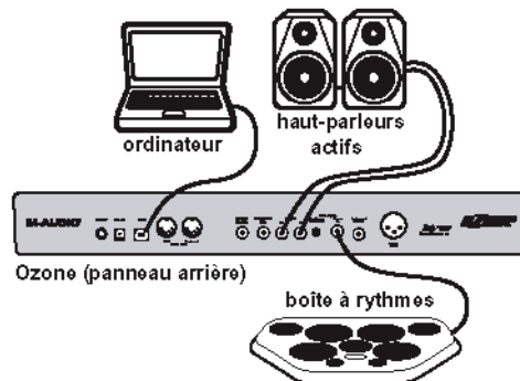
Configuration typique 2
